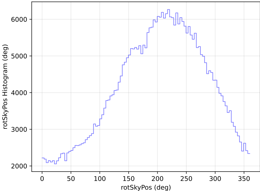
weather_cloudso10v3.4_10yrs All sky y band: rotSkyPos Histogram
