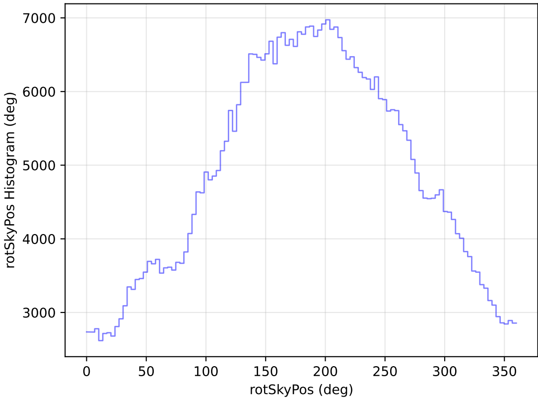
weather_cloudso10v3.4_10yrs All sky r band: rotSkyPos Histogram
