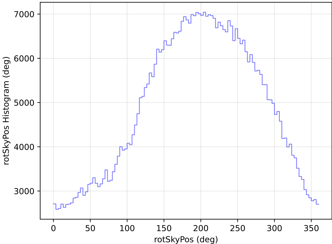
weather_cloudso10v3.4_10yrs All sky i band: rotSkyPos Histogram
