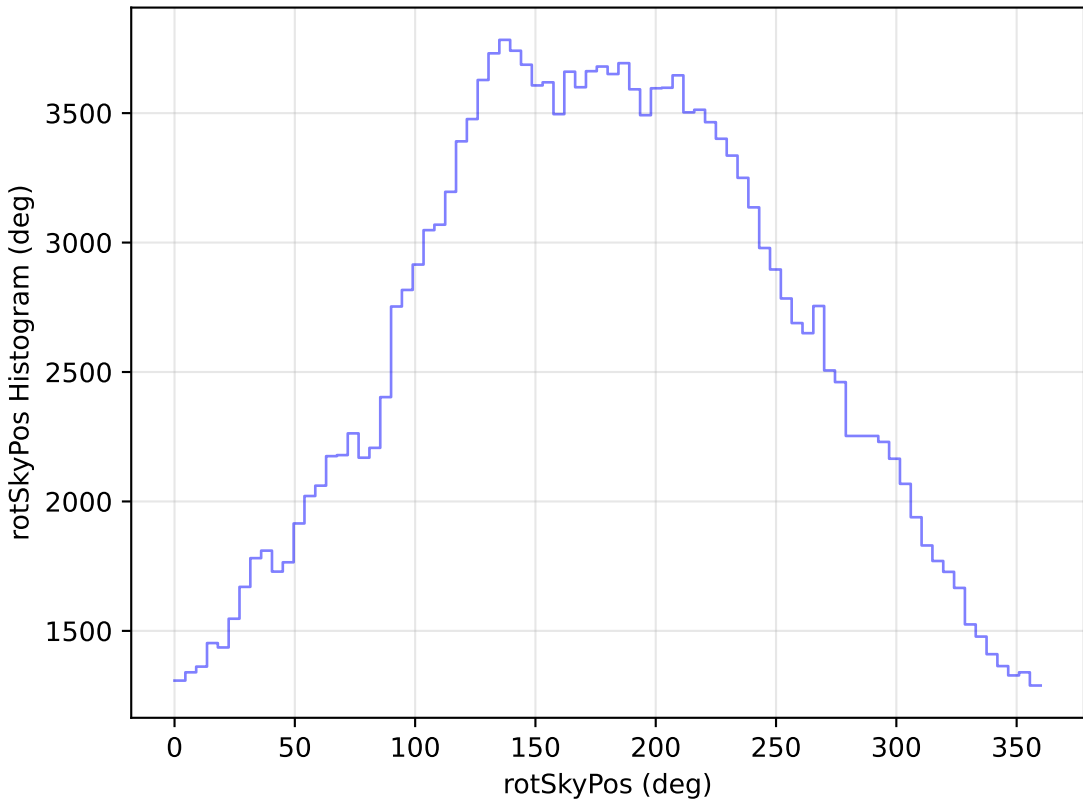
weather_cloudso10v3.4_10yrs All sky g band: rotSkyPos Histogram
