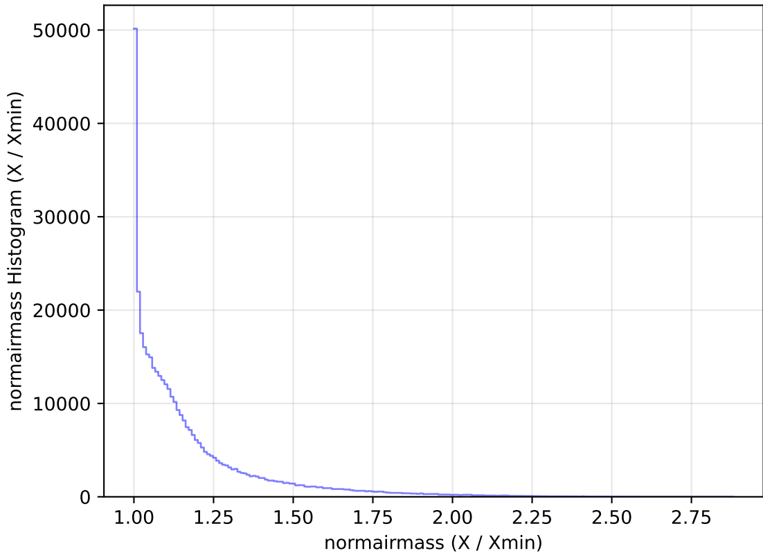
weather_cloudso10v3.4_10yrs WFD y band: normairmass Histogram
