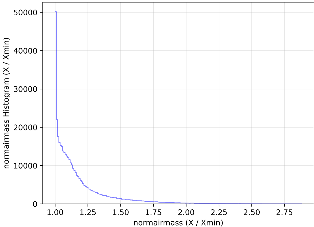
weather_cloudso10v3.4_10yrs All sky y band: normairmass Histogram
