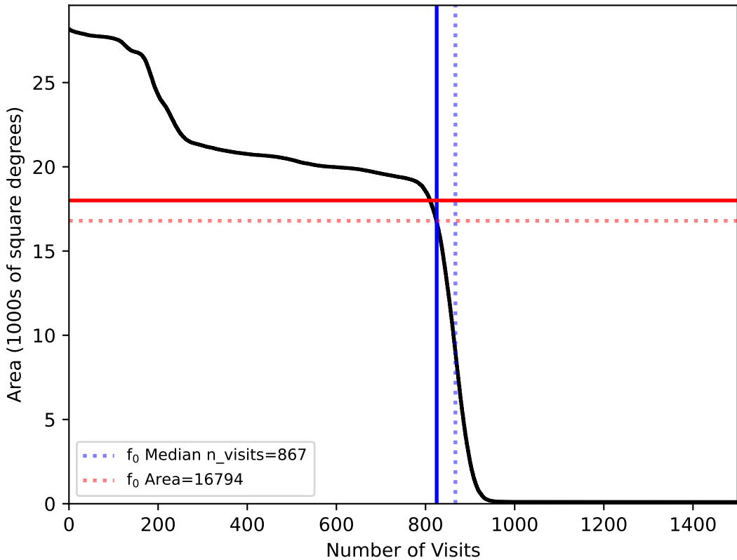
weather_cloudso10v3.4_10yrs All sky: f0
