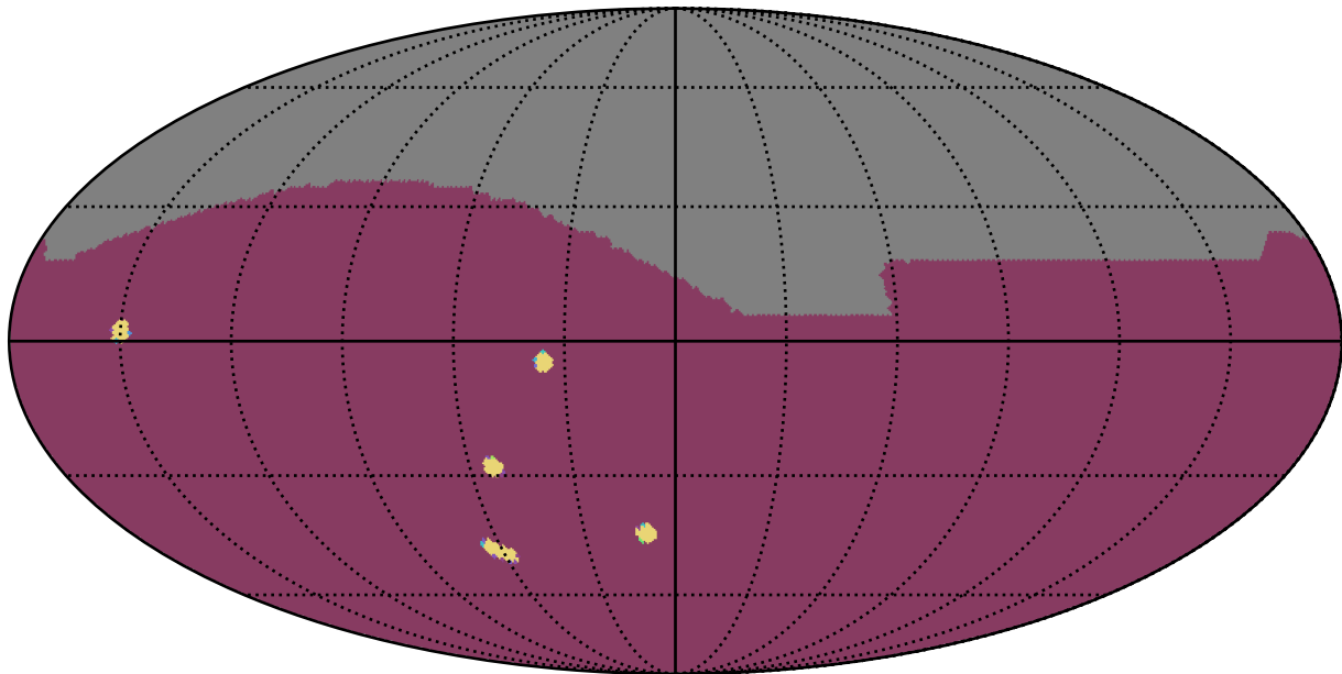
weather_cloudso10v3.4_10yrs All sky: NumberOfQuickRevisits
