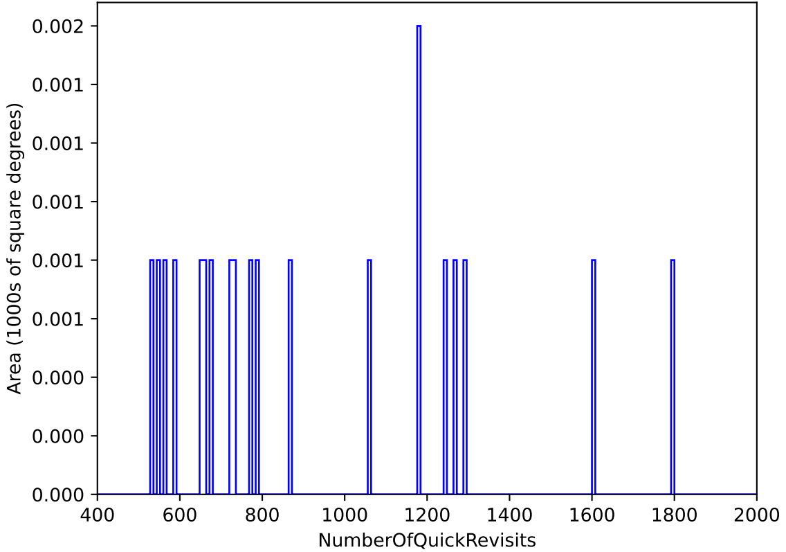
weather_cloudso10v3.4_10yrs All sky: NumberOfQuickRevisits
