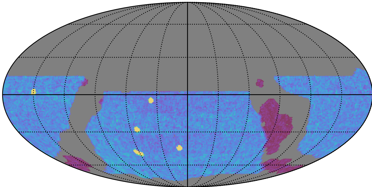
weather_cloudso10v3.4_10yrs WFD y band: NVisits
