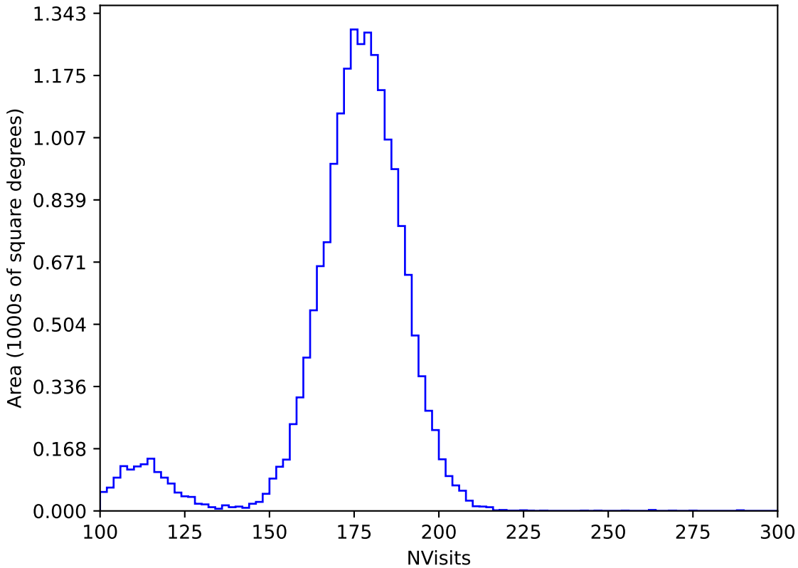
weather_cloudso10v3.4_10yrs WFD y band: NVisits
