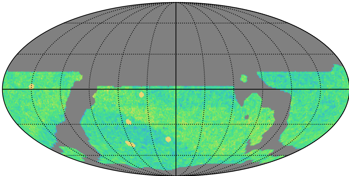
weather_cloudso10v3.4_10yrs WFD i band: NVisits
