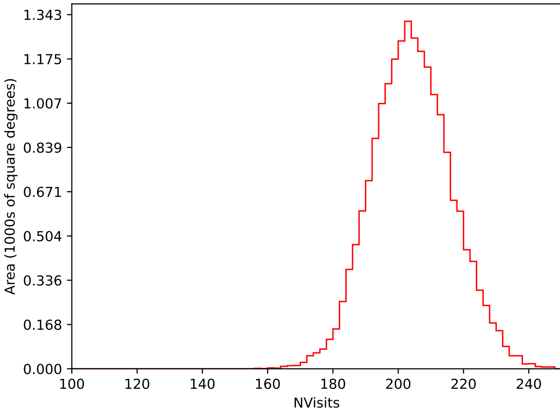
weather_cloudso10v3.4_10yrs WFD i band: NVisits
