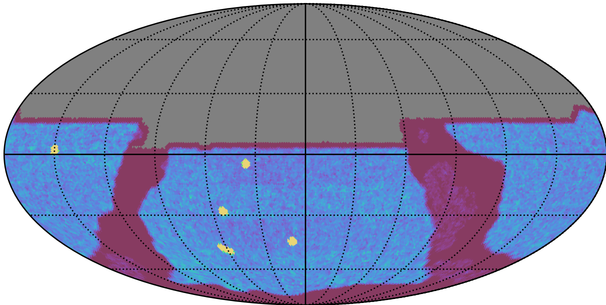
weather_cloudso10v3.4_10yrs All sky y band: NVisits
