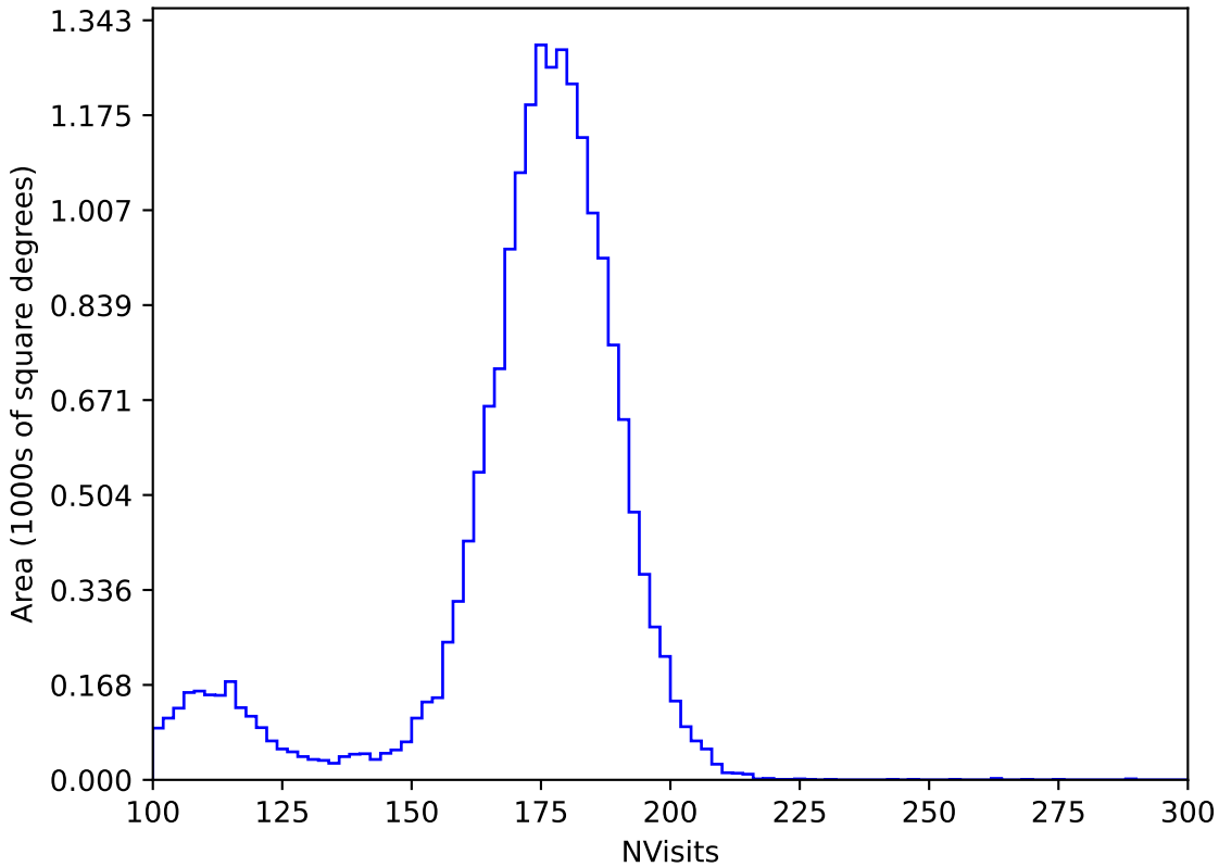
weather_cloudso10v3.4_10yrs All sky y band: NVisits
