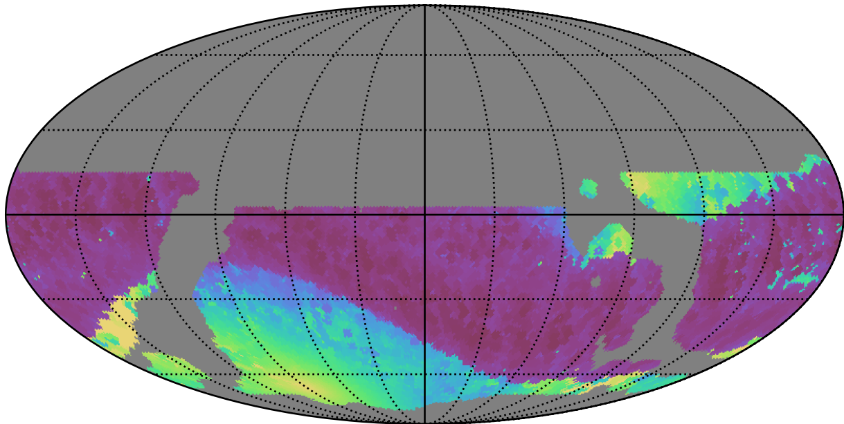
weather_cloudso10v3.4_10yrs WFD z band: Min solarElong
