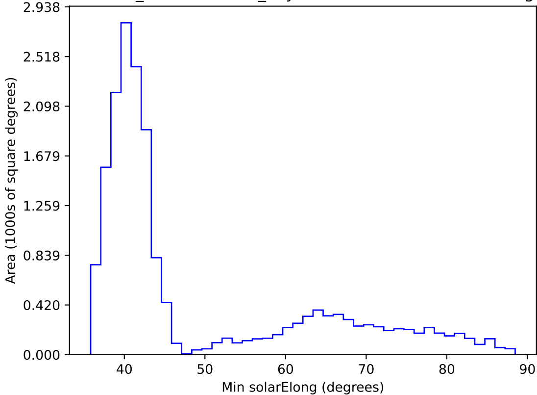
weather_cloudso10v3.4_10yrs WFD z band: Min solarElong
