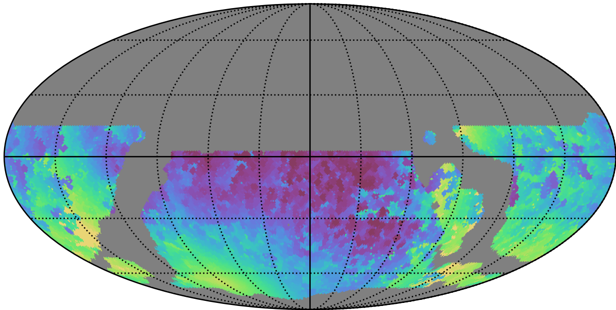
weather_cloudso10v3.4_10yrs WFD y band: Min solarElong
