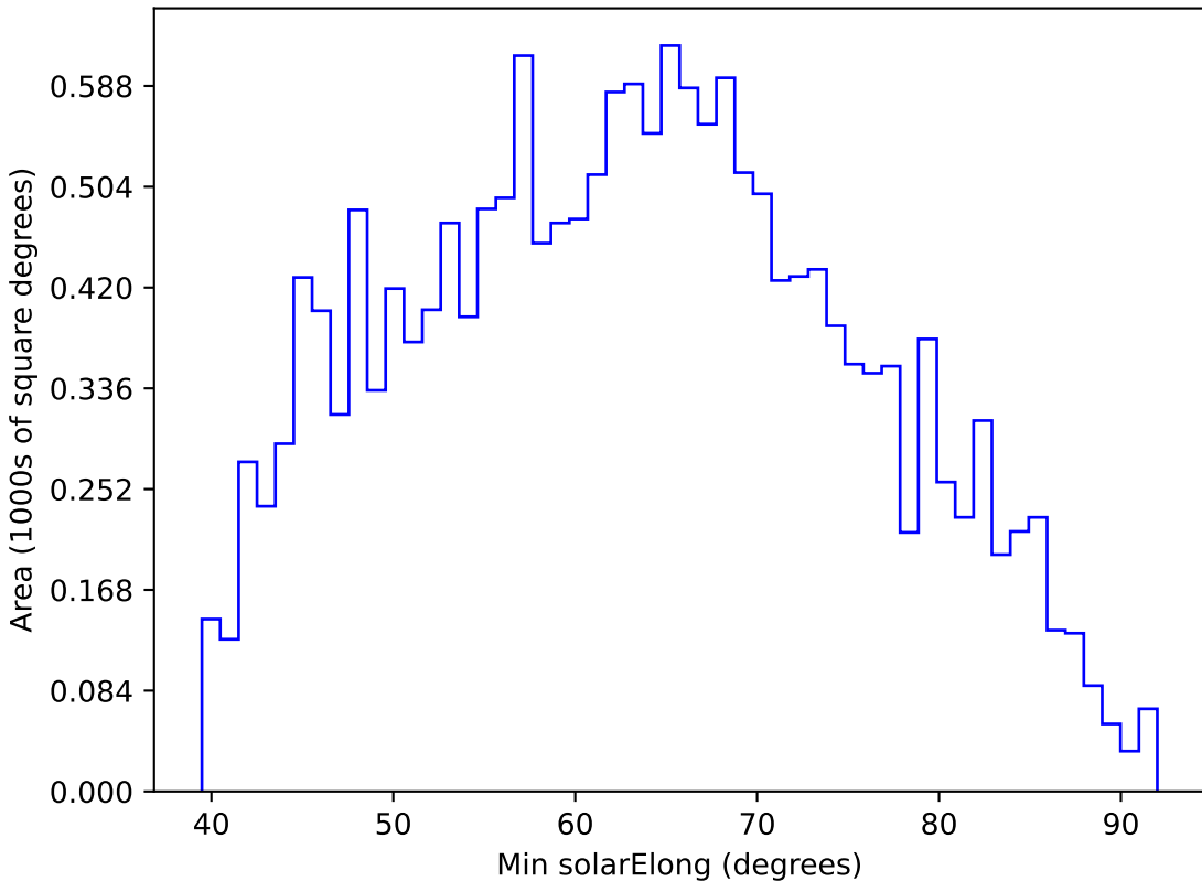
weather_cloudso10v3.4_10yrs WFD y band: Min solarElong
