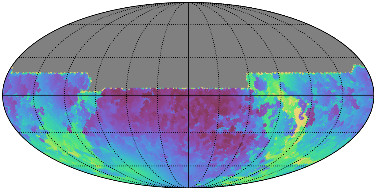
weather_cloudso10v3.4_10yrs All sky y band: Min solarElong
