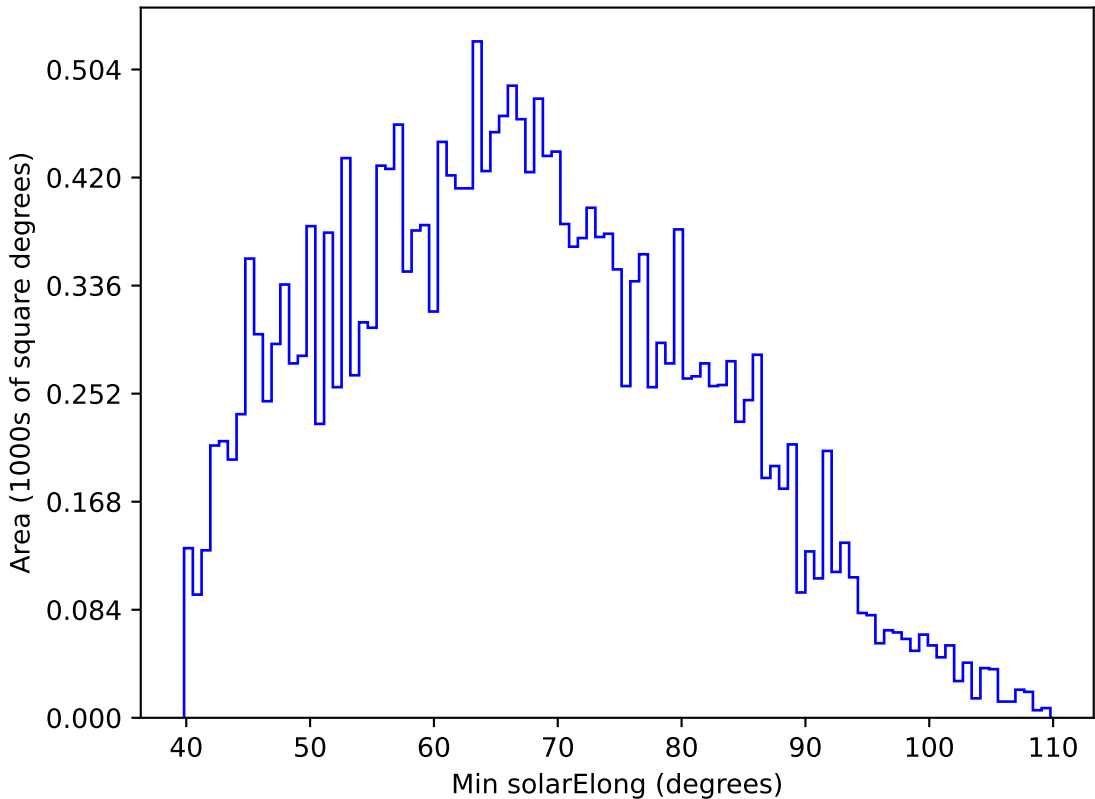
weather_cloudso10v3.4_10yrs All sky y band: Min solarElong
