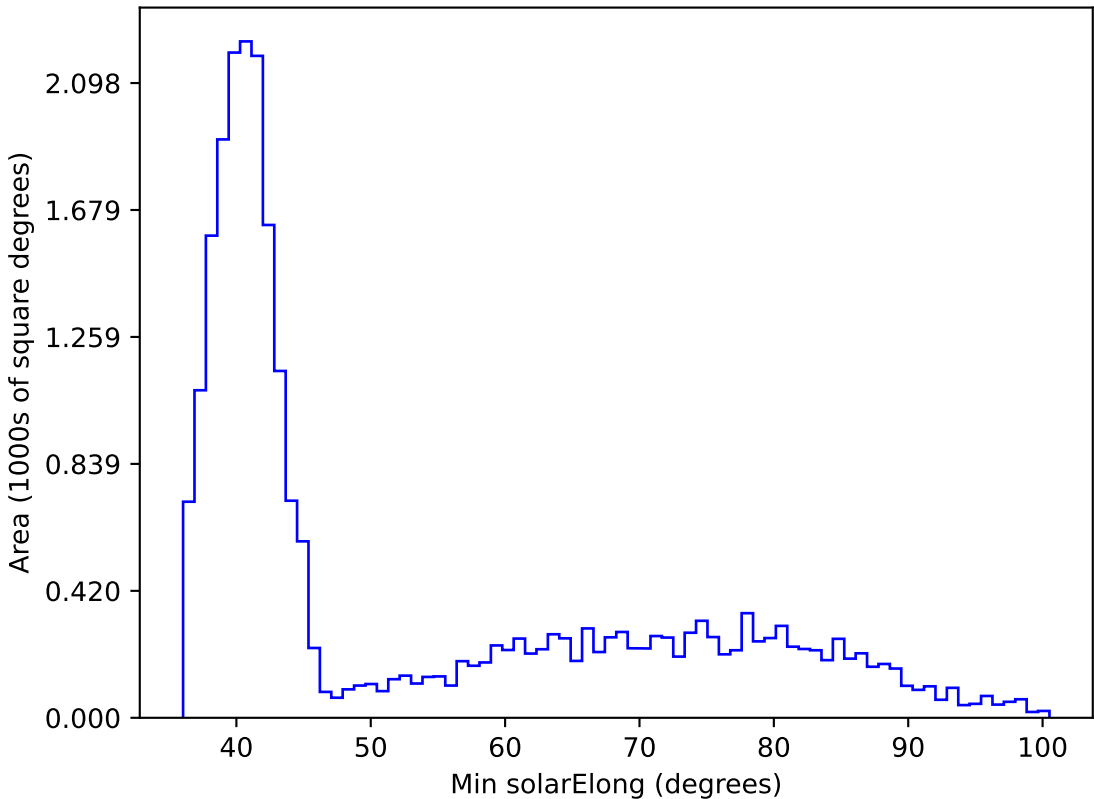
weather_cloudso10v3.4_10yrs All sky i band: Min solarElong
