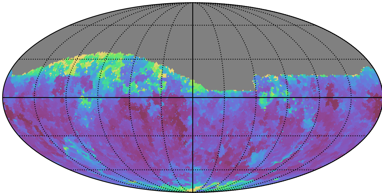
weather_cloudso10v3.4_10yrs Yr 1 z band: Min seeingGeom
