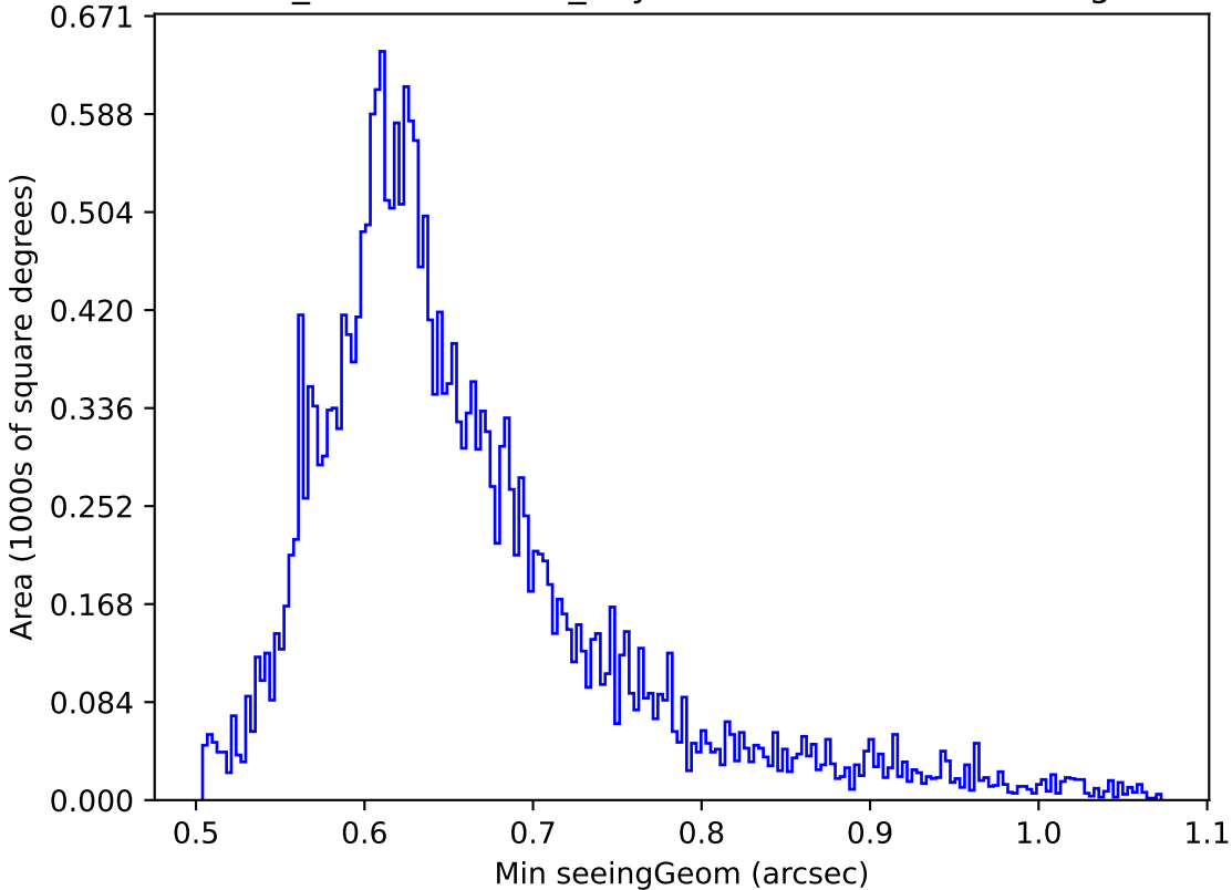
weather_cloudso10v3.4_10yrs Yr 1 z band: Min seeingGeom
