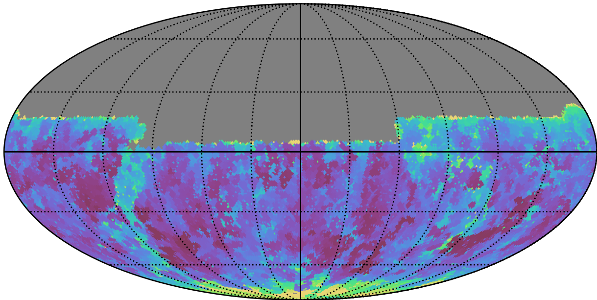
weather_cloudso10v3.4_10yrs Yr 1 y band: Min seeingGeom
