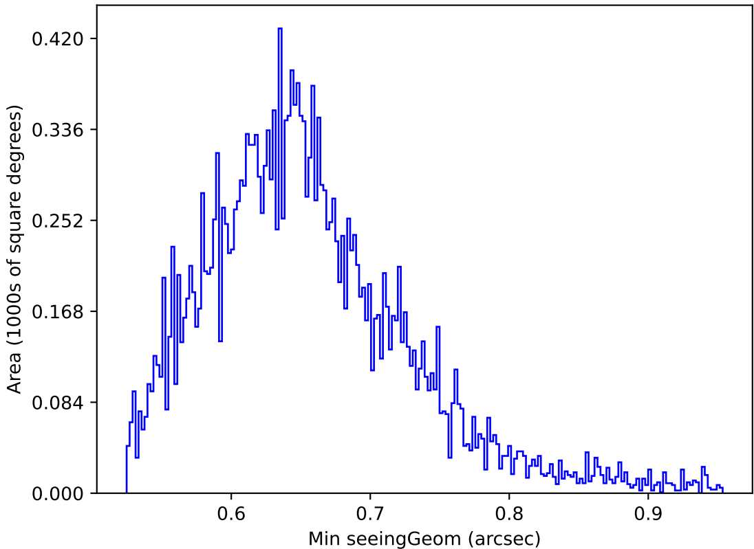
weather_cloudso10v3.4_10yrs Yr 1 y band: Min seeingGeom
