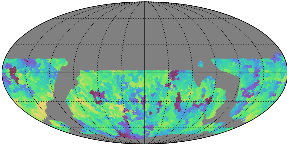
weather_cloudso10v3.4_10yrs WFD z band: Min saturation_mag
