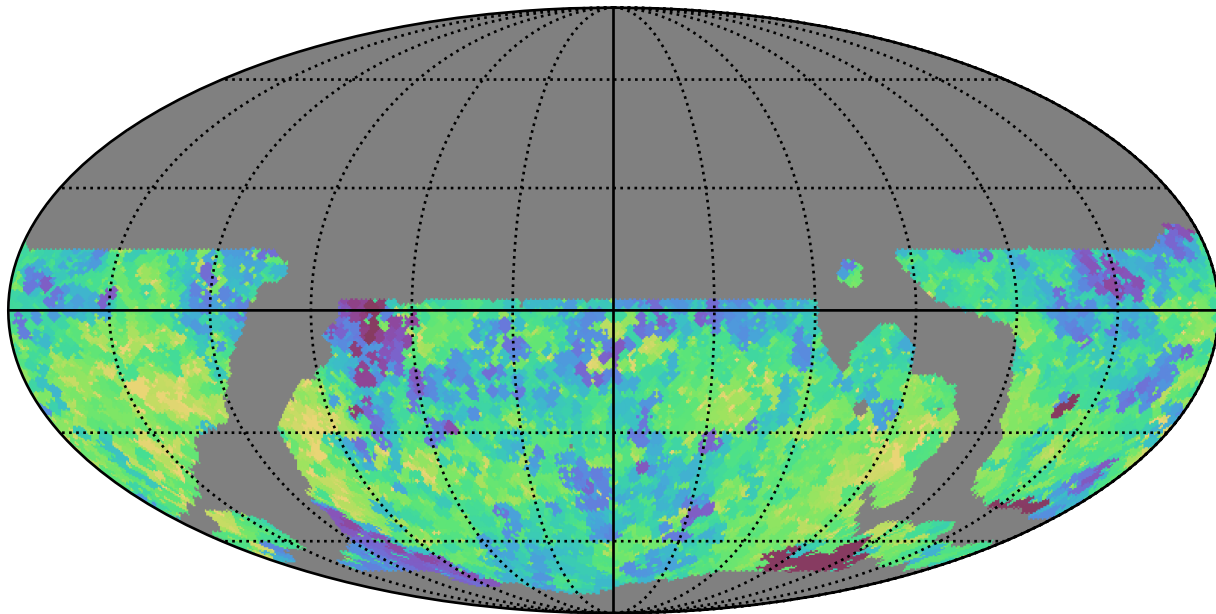
weather_cloudso10v3.4_10yrs WFD y band: Min saturation_mag
