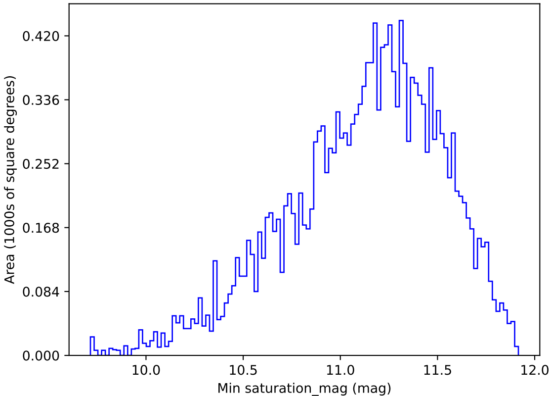
weather_cloudso10v3.4_10yrs WFD y band: Min saturation_mag
