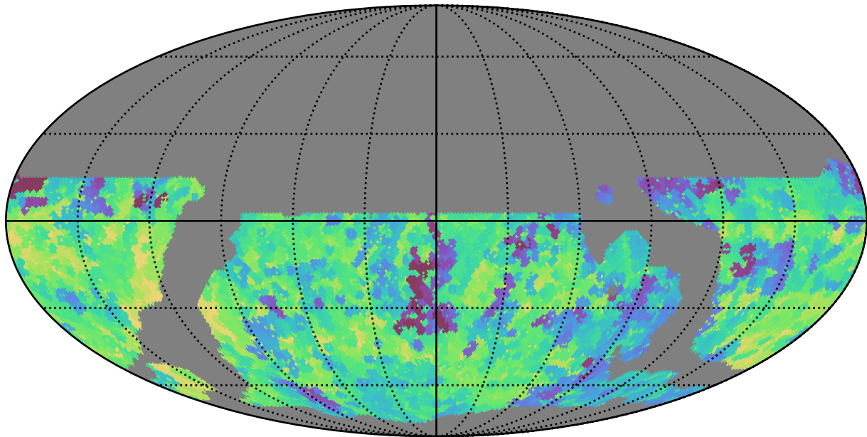
weather_cloudso10v3.4_10yrs WFD r band: Min saturation_mag
