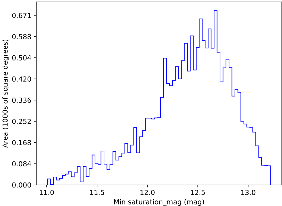
weather_cloudso10v3.4_10yrs WFD r band: Min saturation_mag
