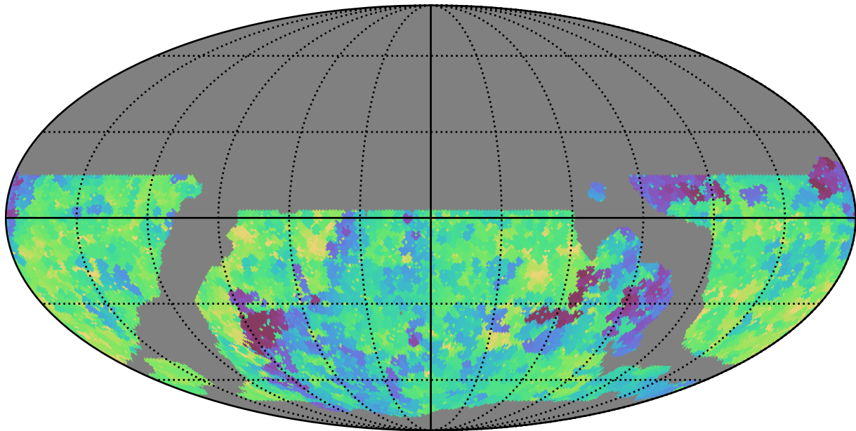
weather_cloudso10v3.4_10yrs WFD g band: Min saturation_mag
