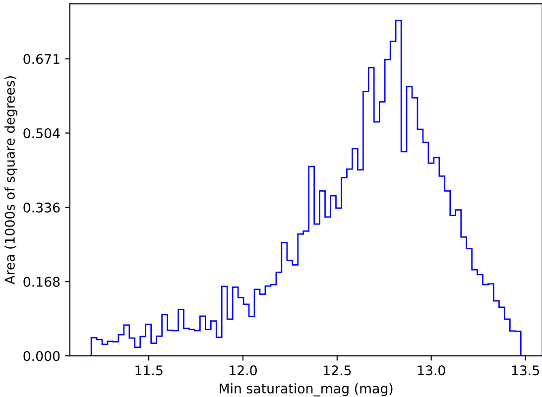
weather_cloudso10v3.4_10yrs WFD g band: Min saturation_mag
