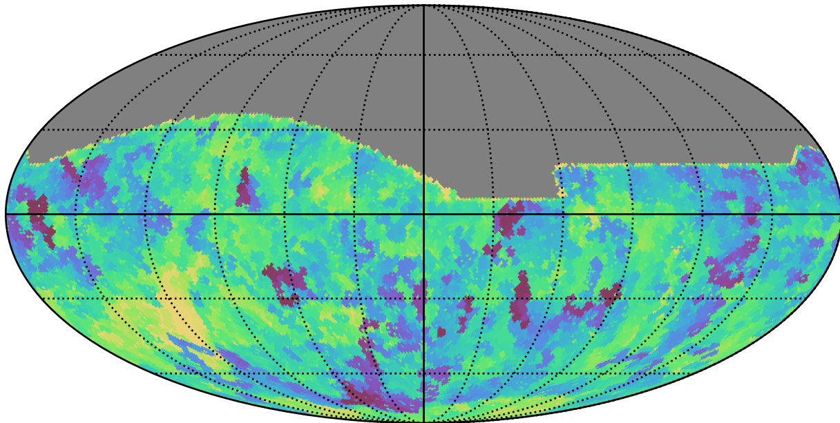
weather_cloudso10v3.4_10yrs All sky z band: Min saturation_mag
