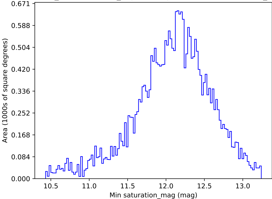
weather_cloudso10v3.4_10yrs All sky z band: Min saturation_mag
