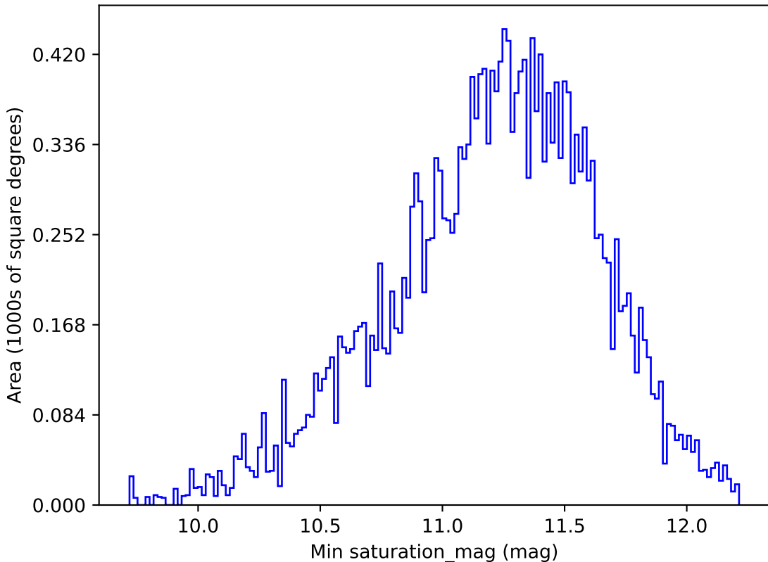
weather_cloudso10v3.4_10yrs All sky y band: Min saturation_mag
