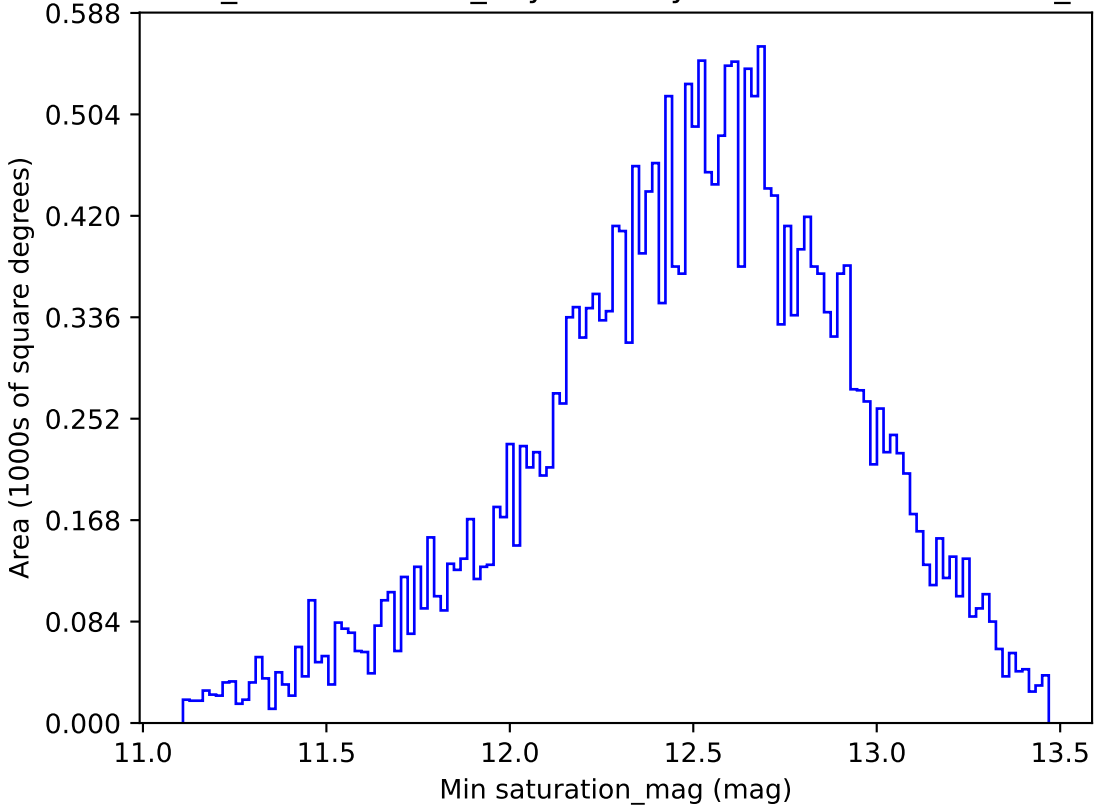
weather_cloudso10v3.4_10yrs All sky r band: Min saturation_mag
