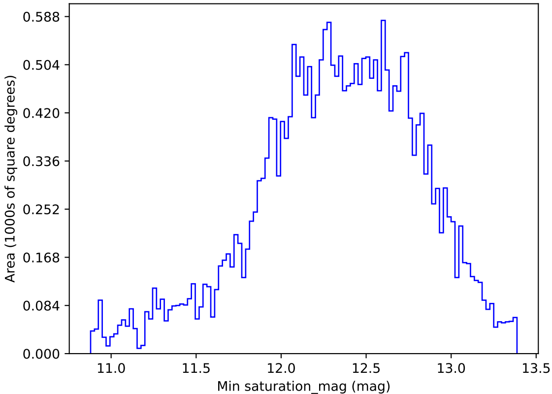
weather_cloudso10v3.4_10yrs All sky i band: Min saturation_mag
