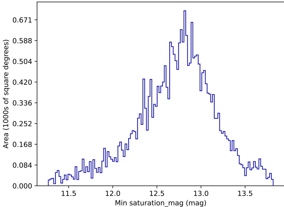
weather_cloudso10v3.4_10yrs All sky g band: Min saturation_mag
