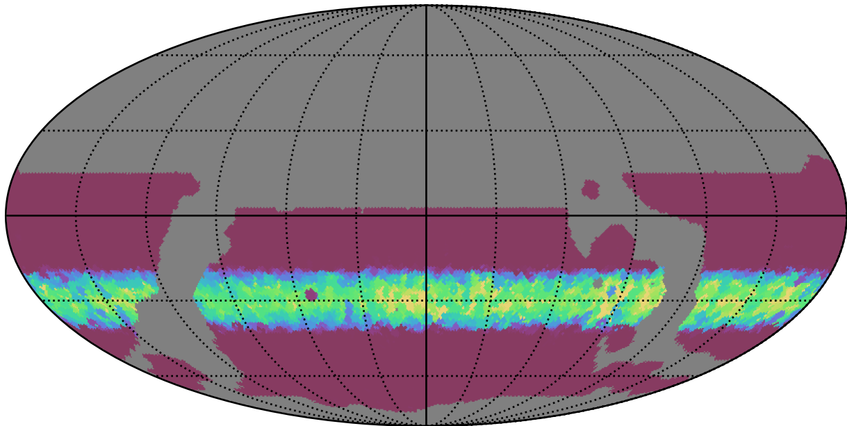
weather_cloudso10v3.4_10yrs WFD z band: Min normairmass
