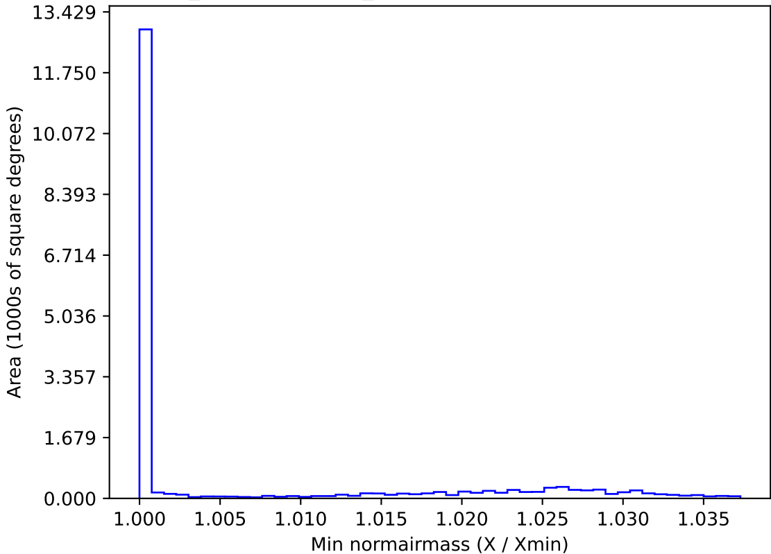
weather_cloudso10v3.4_10yrs WFD z band: Min normairmass
