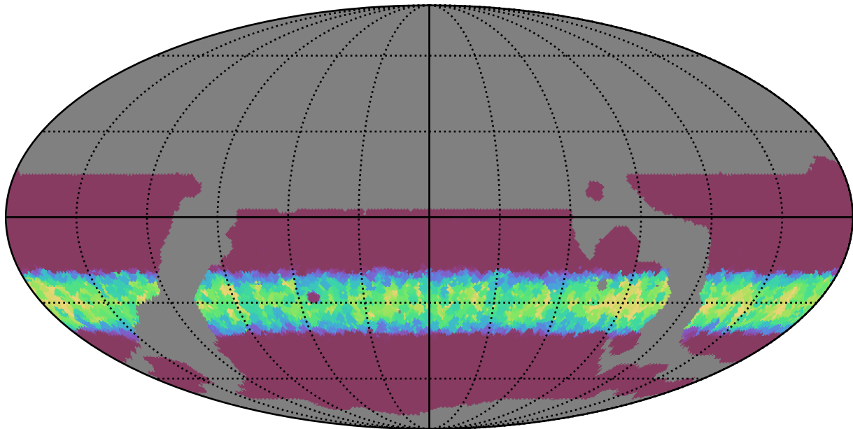
weather_cloudso10v3.4_10yrs WFD y band: Min normairmass
