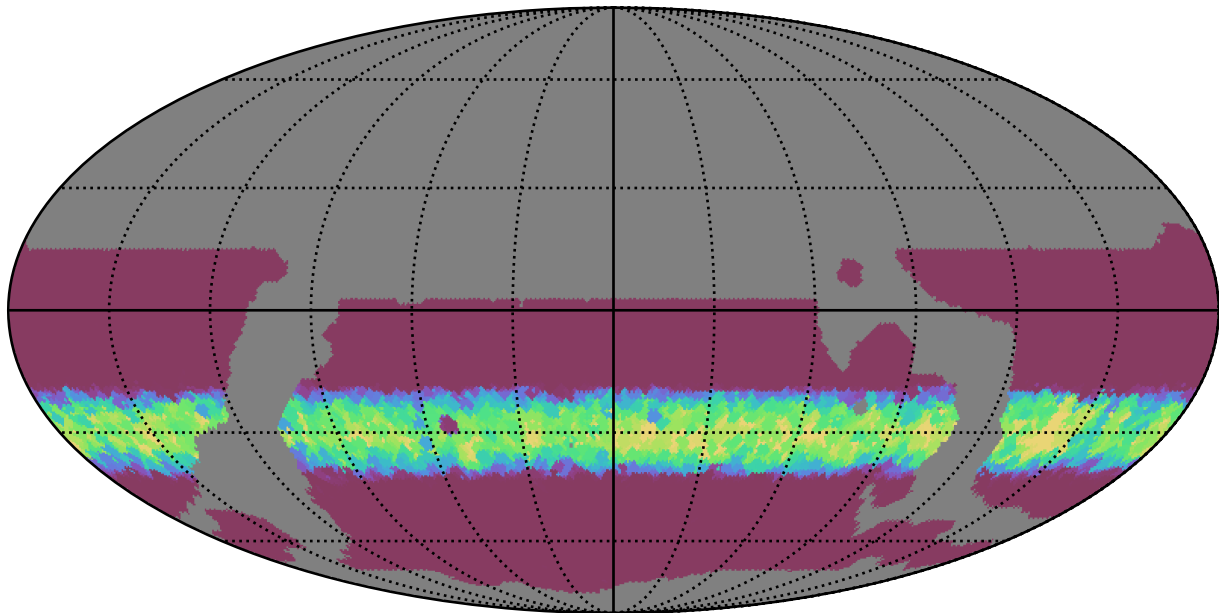
weather_cloudso10v3.4_10yrs WFD i band: Min normairmass
