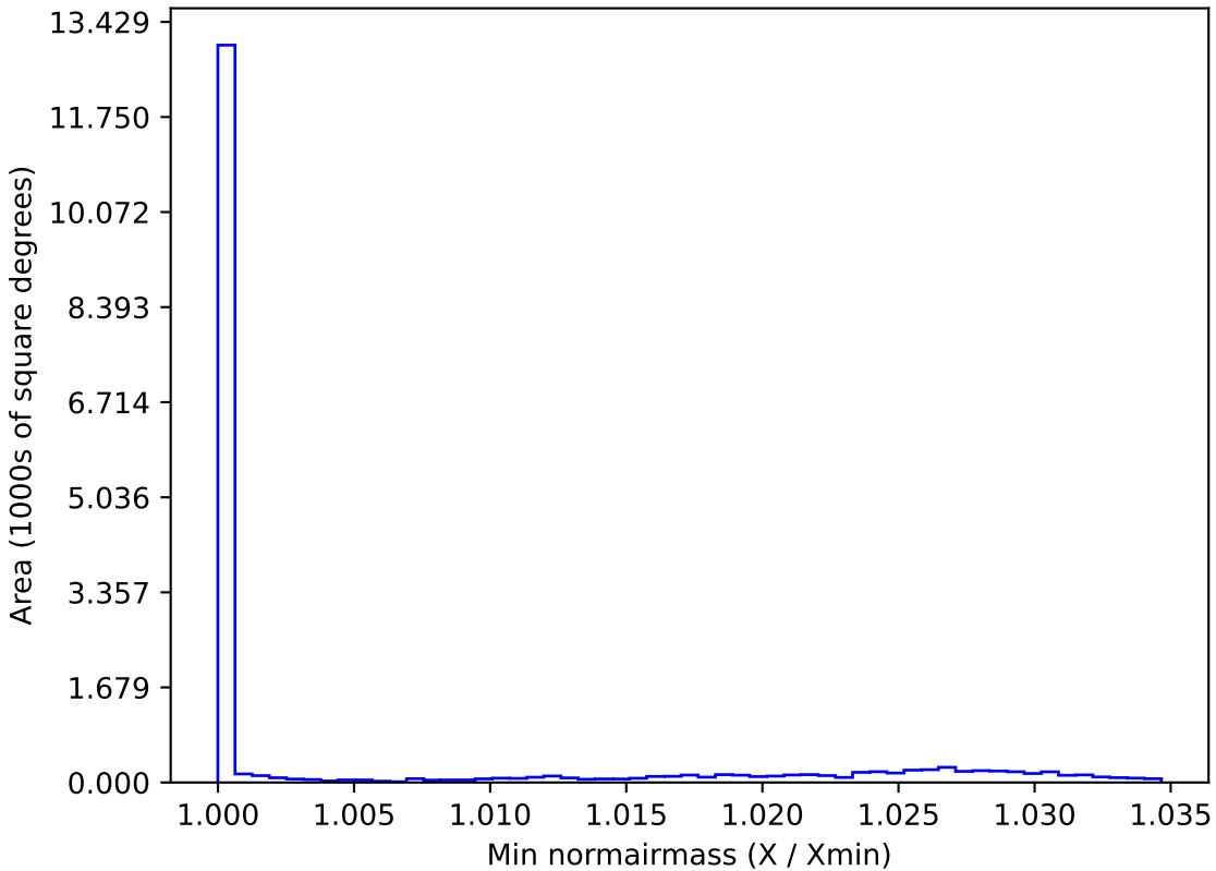
weather_cloudso10v3.4_10yrs WFD i band: Min normairmass
