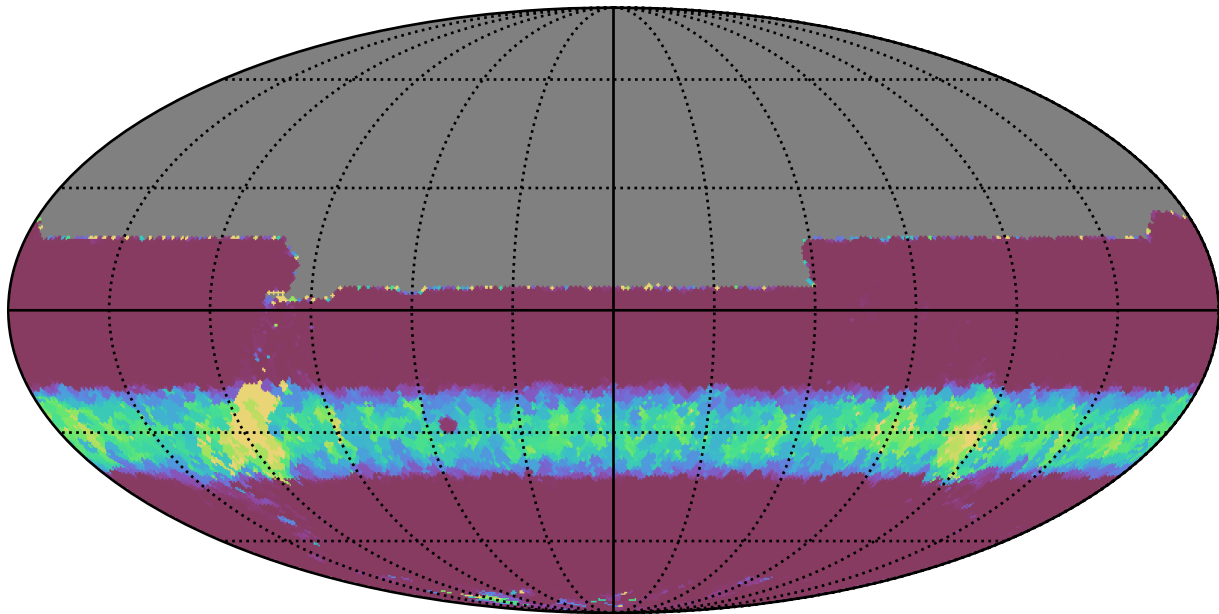
weather_cloudso10v3.4_10yrs All sky y band: Min normairmass
