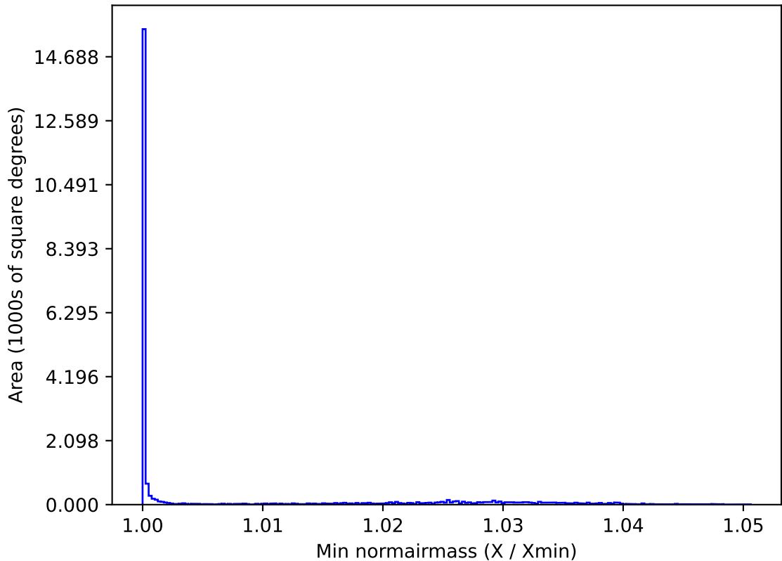
weather_cloudso10v3.4_10yrs All sky y band: Min normairmass
