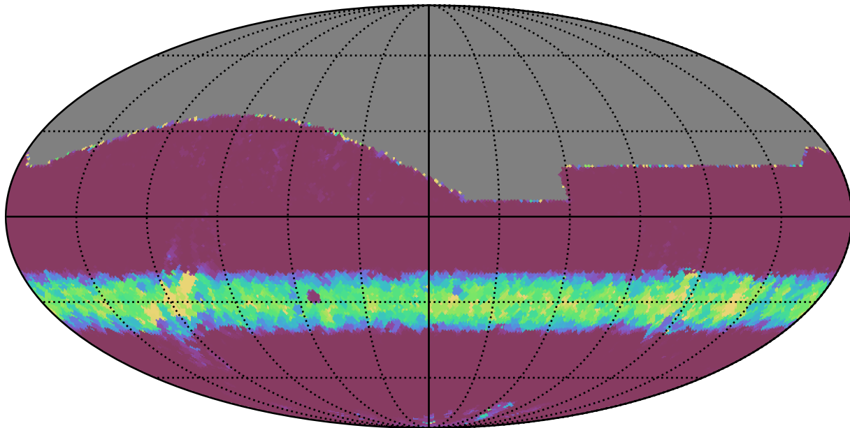
weather_cloudso10v3.4_10yrs All sky i band: Min normairmass
