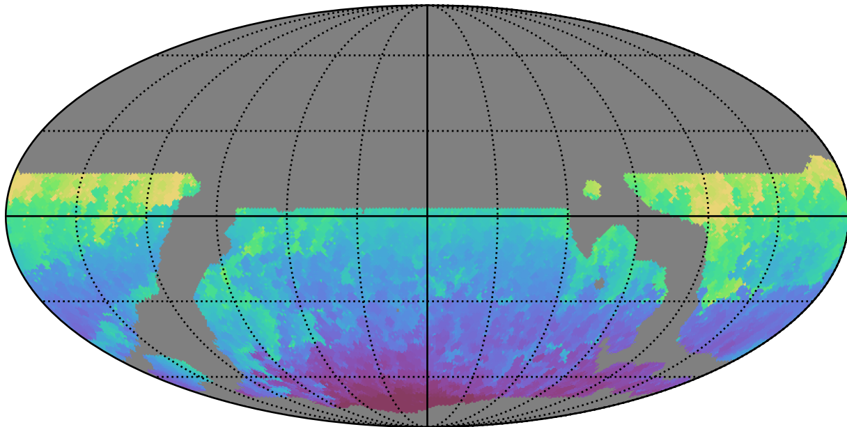
weather_cloudso10v3.4_10yrs WFD z band: Min HA
