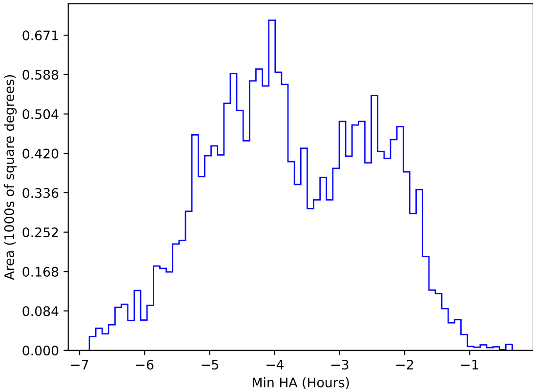
weather_cloudso10v3.4_10yrs WFD y band: Min HA
