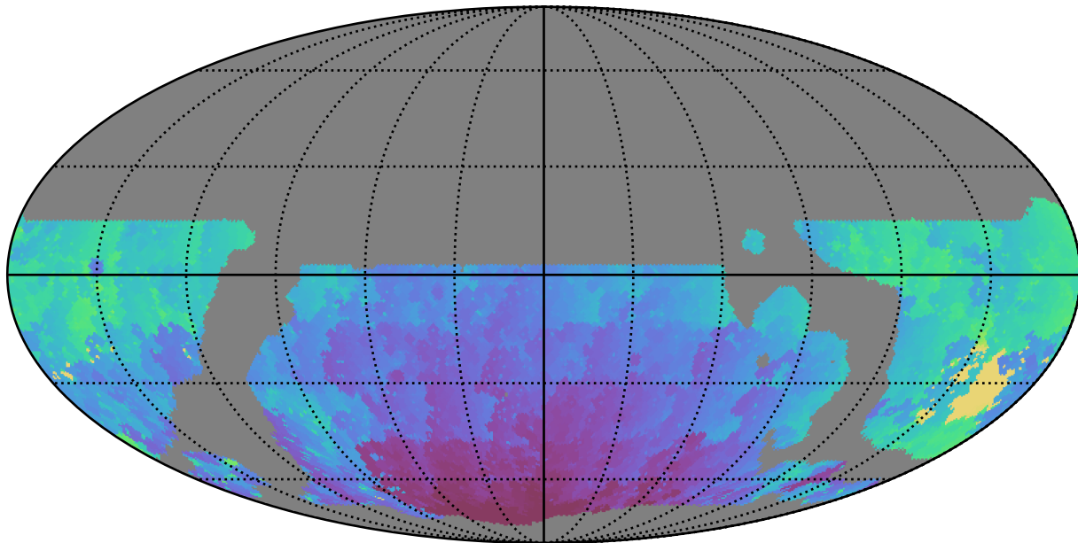
weather_cloudso10v3.4_10yrs WFD u band: Min HA
